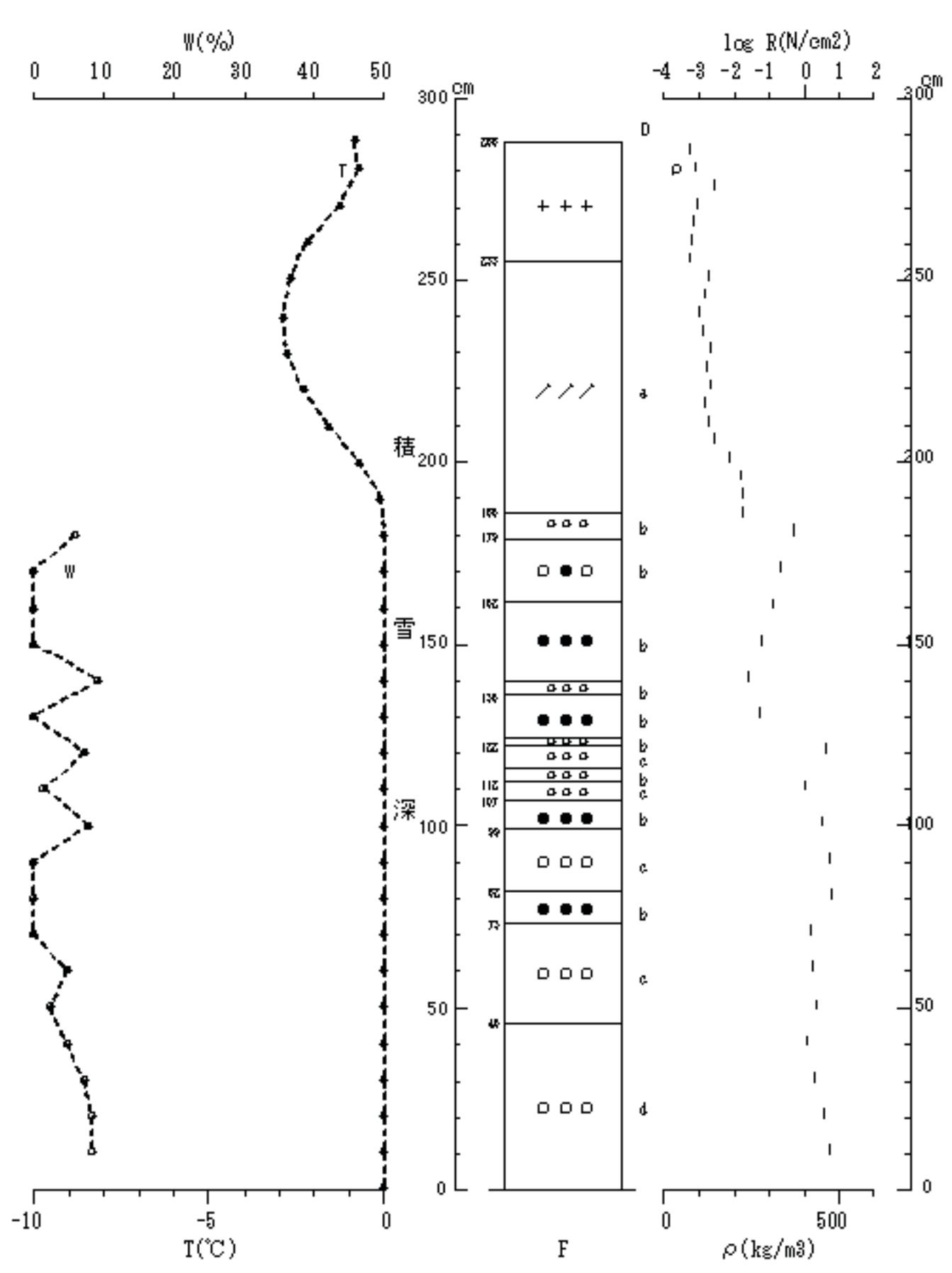
図 No. 積雪断面観測結果 ( '2010/01/15 山古志種芋原 )
