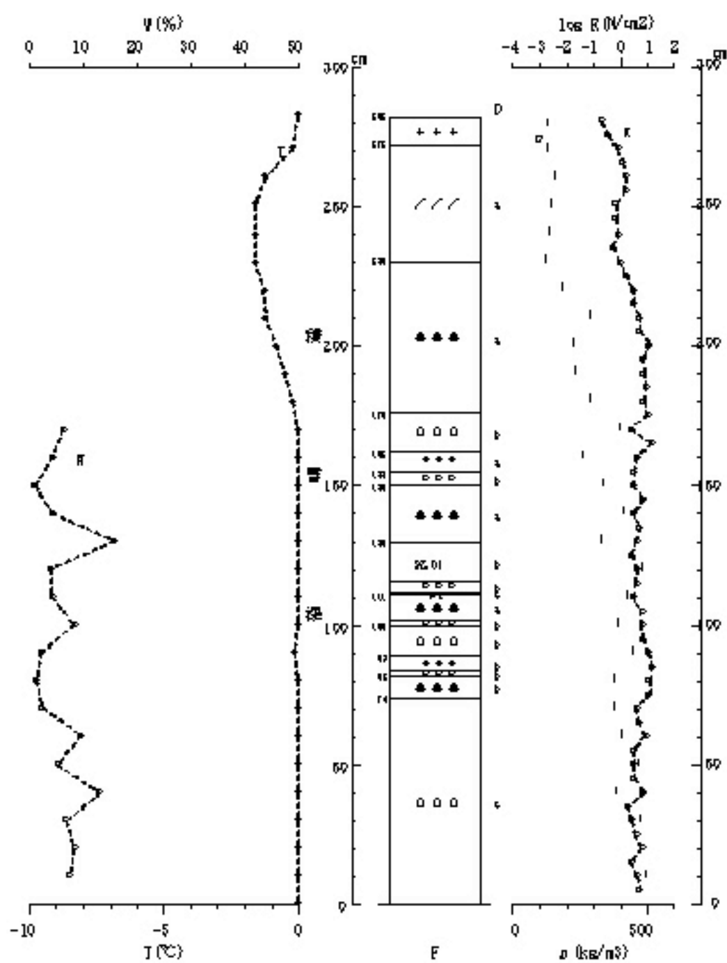
図 No. 積雪断面観測結果 ( '2010/01/18 山古志種芋原 )
