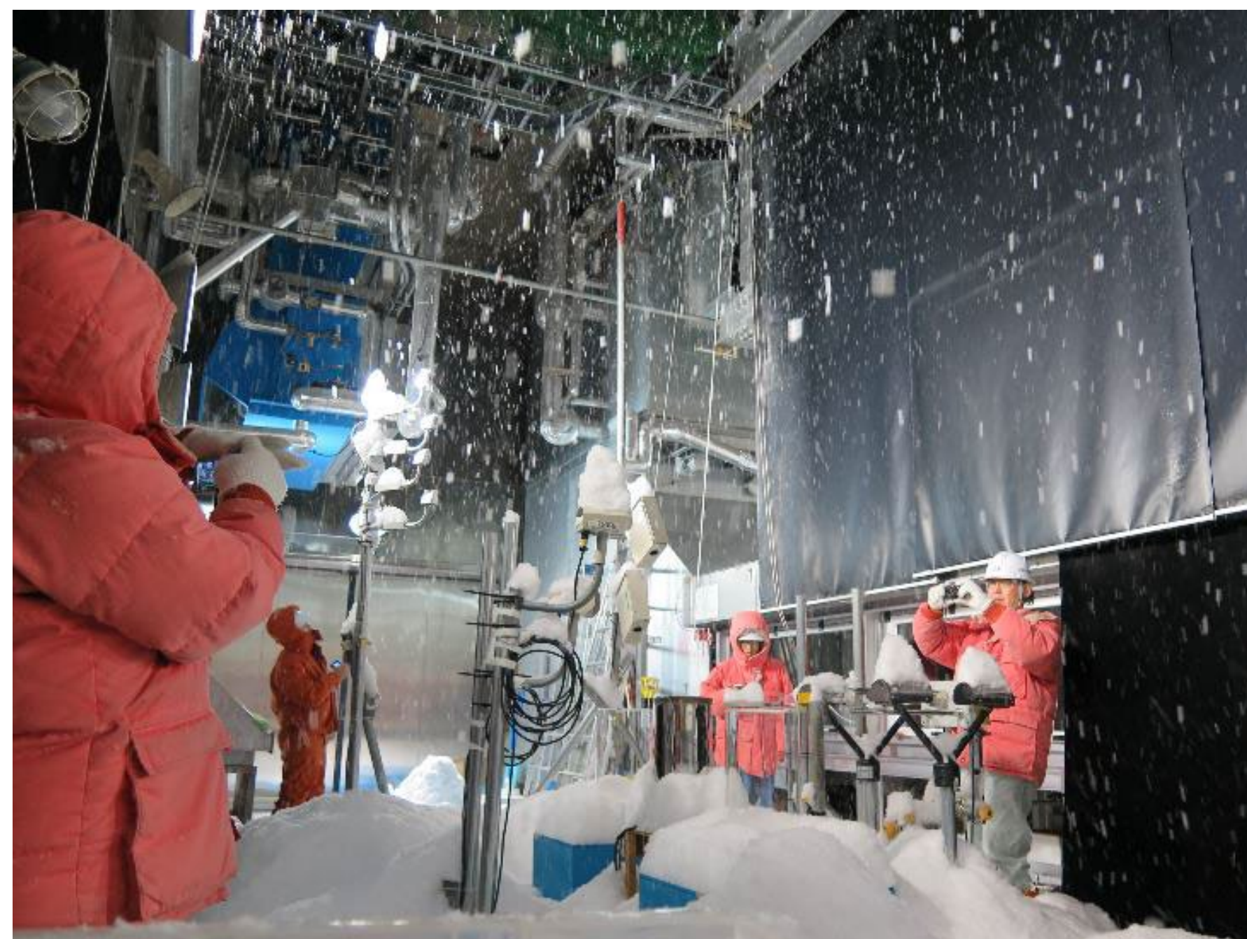
図2 新型降雪・積雪センサーの開発（長岡技術科学大学との共同研究）
