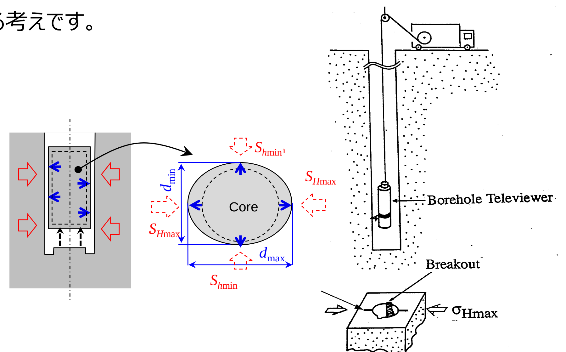
左図、コア変形法の原理。掘削直後、応力解放により岩石コアが弾性変形し、コア断面が水平最大圧縮応力( S_{Hmax} )の方向に扁平な楕円状になる。 右図、ボアホールブレイクアウト法の原理。掘削直後、応力集中によりせん断破壊し、水平最大圧縮応力( S_{Hmax} )から90°の方向の孔壁の一部が崩壊する。
