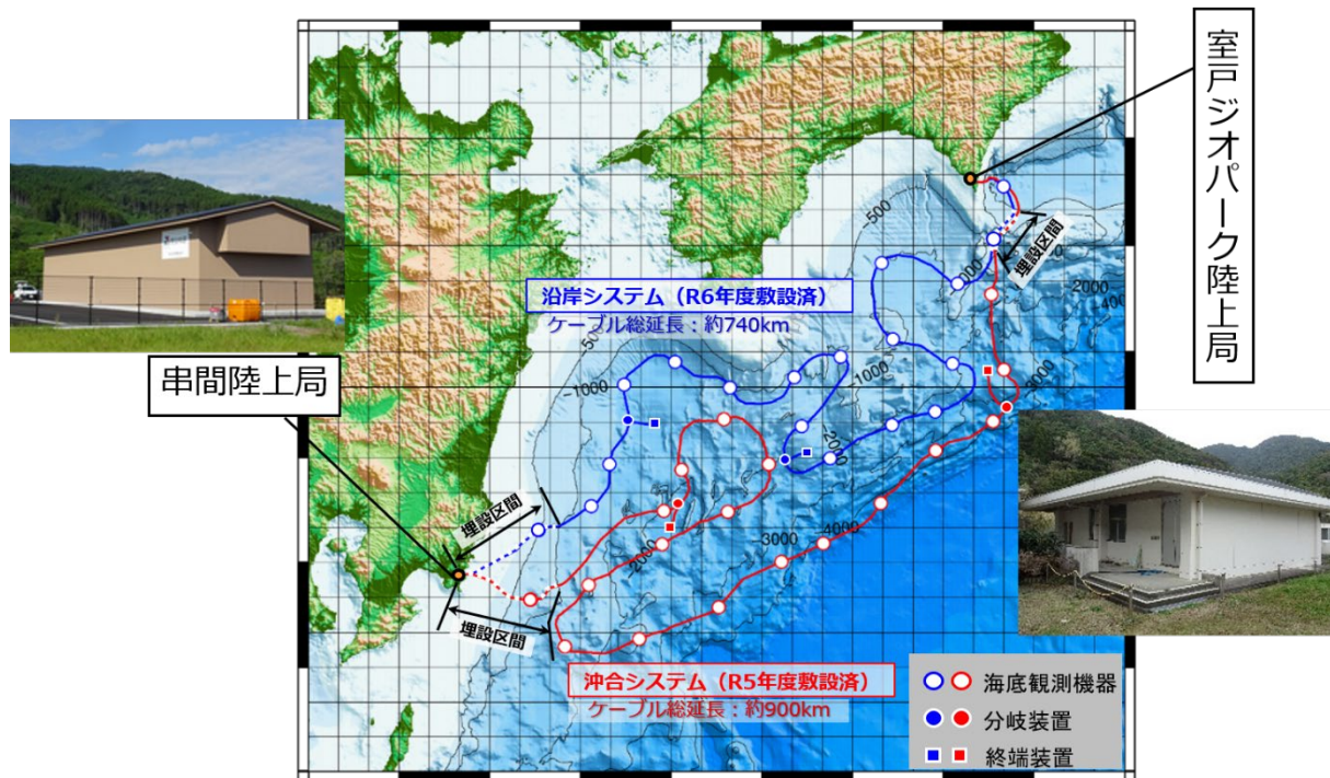
図 N-net 観測点配置図
